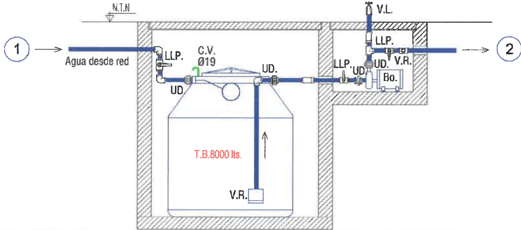
TANQUE CISTERNA - VISTA EN CORTE
