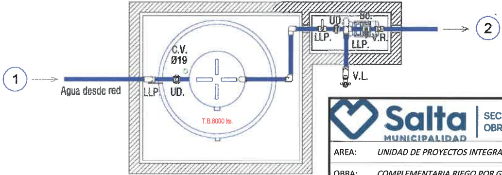
TANQUE CISTERNA - VISTA EN PLANTA
