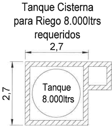
DETALLE CISTERNA TIPO - ESC. S/E
