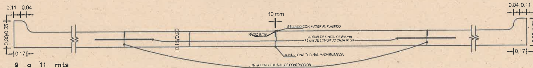
SECCIONES TRANSVERSALES DE CALZADA Y CORDON
