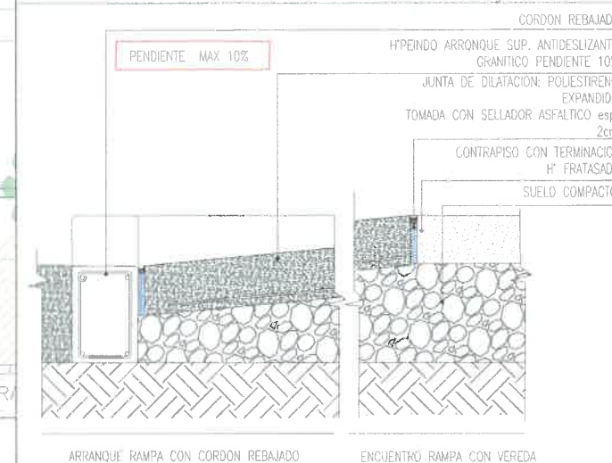
DO3-RAMPA ACCESIBILIDAD
