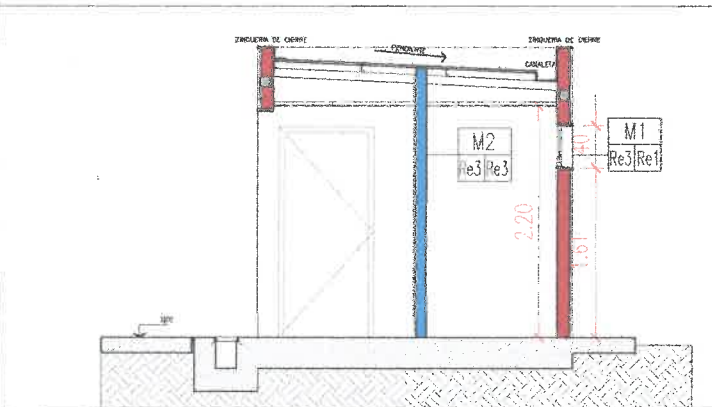
ESQUEMA ESTRUCTURAL DE CUBIERTA MODULO - ESC. 1:50
