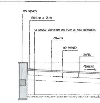
D02-ENCUENTRO TECHO MODULO SANITARIO
