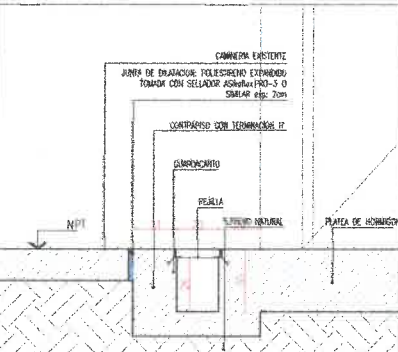
D01-REJILLA DE DESAGUE PLUVIAL
