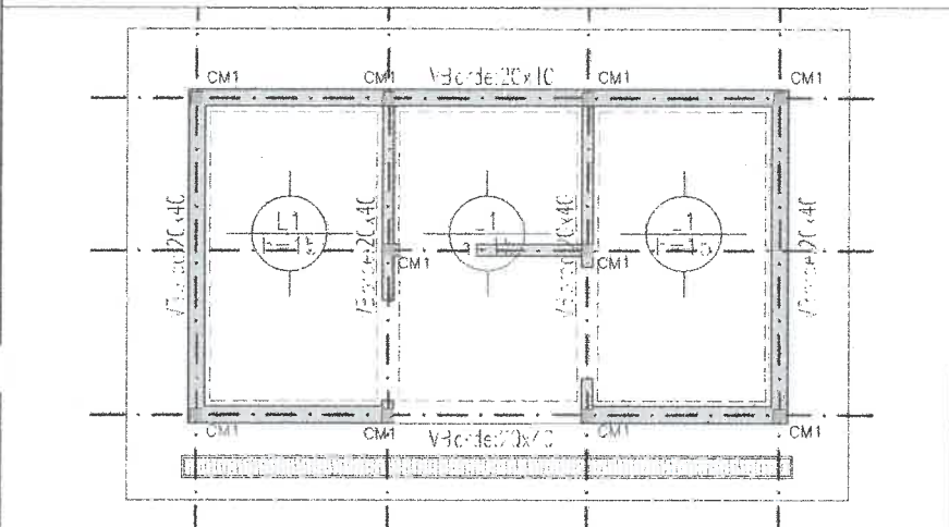
BASE ESTRUCTURAL MODULO SANITARIO - ESC. 1:50
