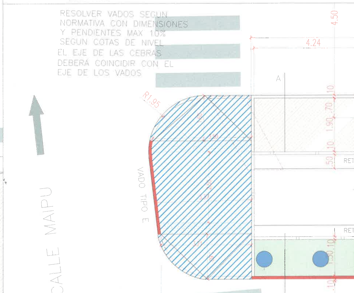
VADO TIPO E ESC. 1:75
