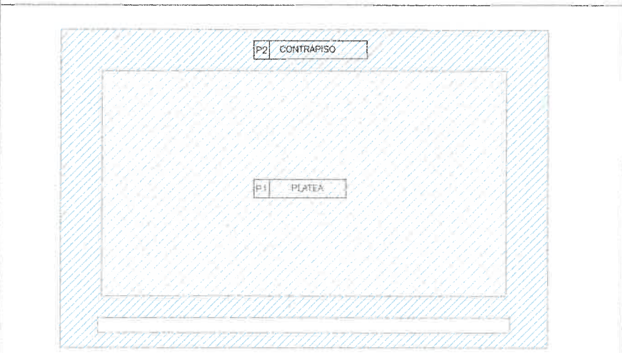
BASE ESTRUCTURAL MODULO SANITARIO - ESC. 1:50
