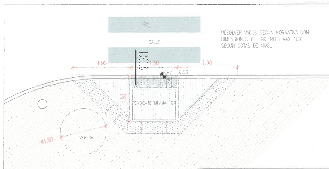
VADO TIPO B ESC. 1:75
