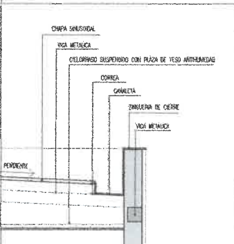
D03-ENCUENTRO TECHO MODULO SANITARIO
