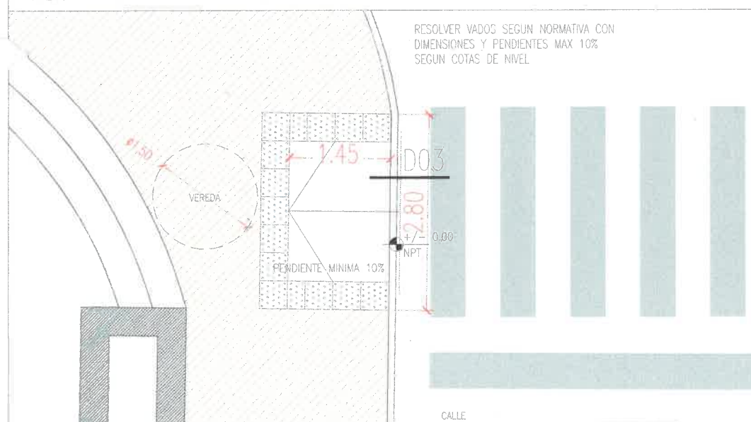
VADO TIPO C ESC. 1:75
