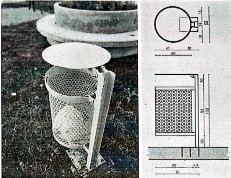
Imagen ilustrativa del cesto y detalle constructivo
