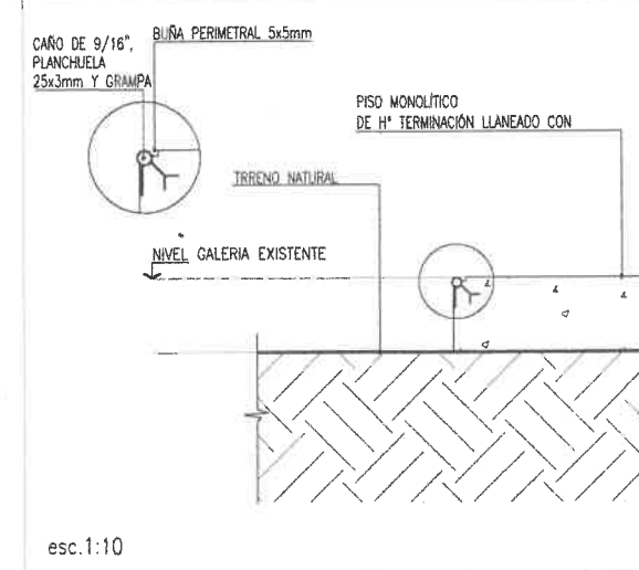
D03-PLANCHUELA EN GALERIA
