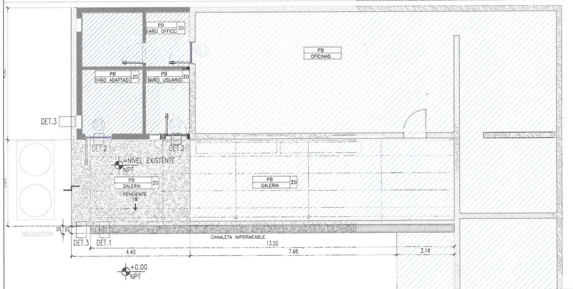
D01-CANALETA IMPERMEABLE
