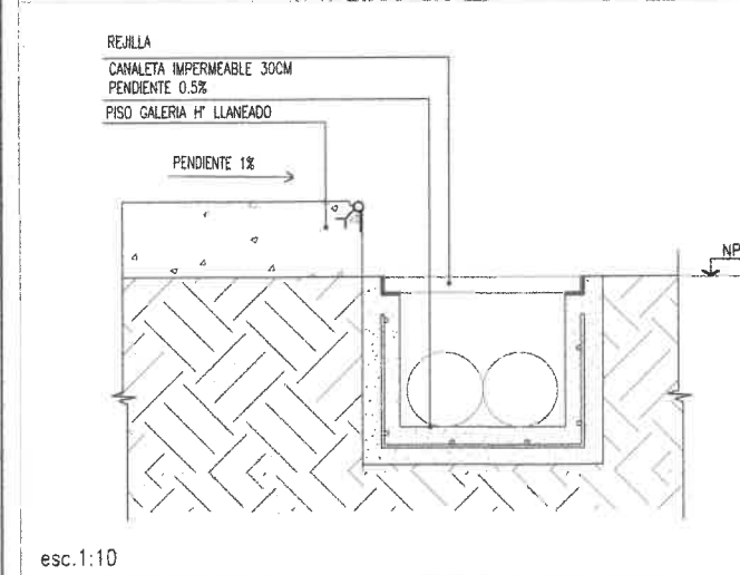
D01-CANALETA IMPERMEABLE
