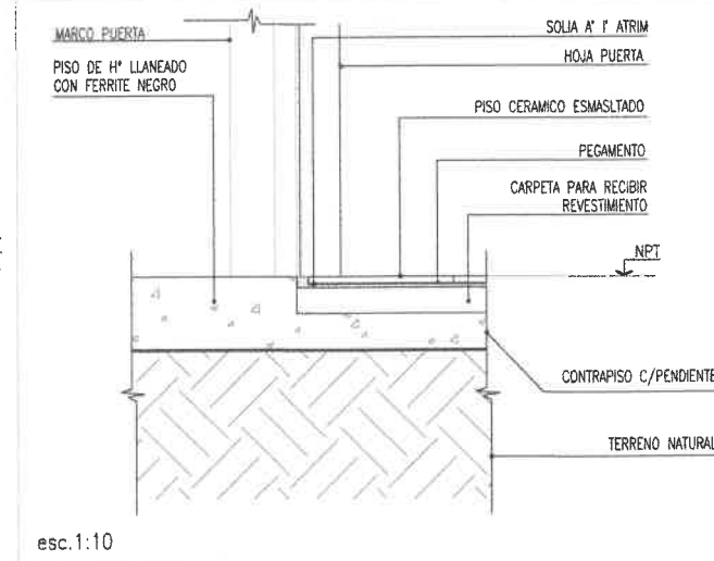
D02-ENCUENTRO SOLADO SANITARIOS Y GALERIA
