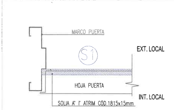
DETALLE POSICIÓN DE SOLIA
