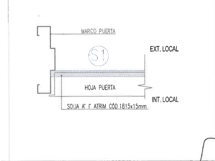
DETALLE POSICIÓN DE SOLIA
